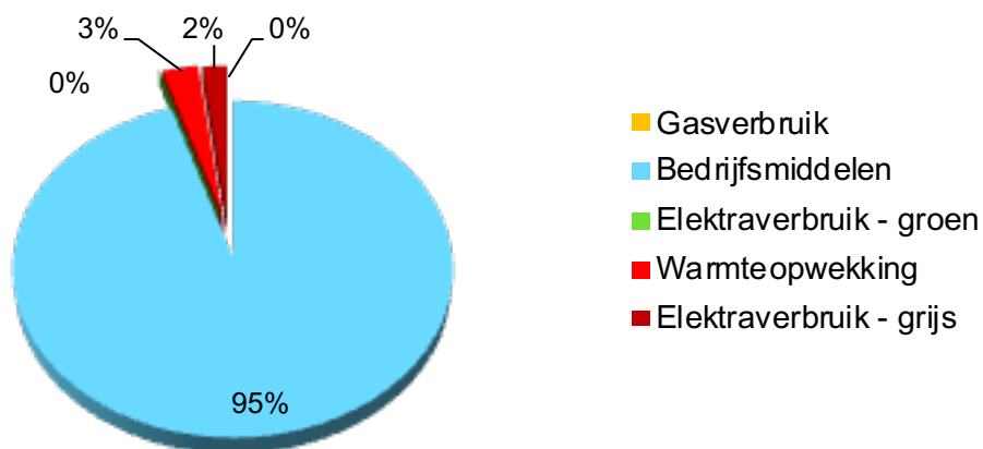
Scope 1 en 2 emissies van Groen Beheer Grafhorst (totaal = 2.230 ton CO 2 )
